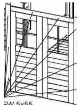
木ネジで前面から固定
