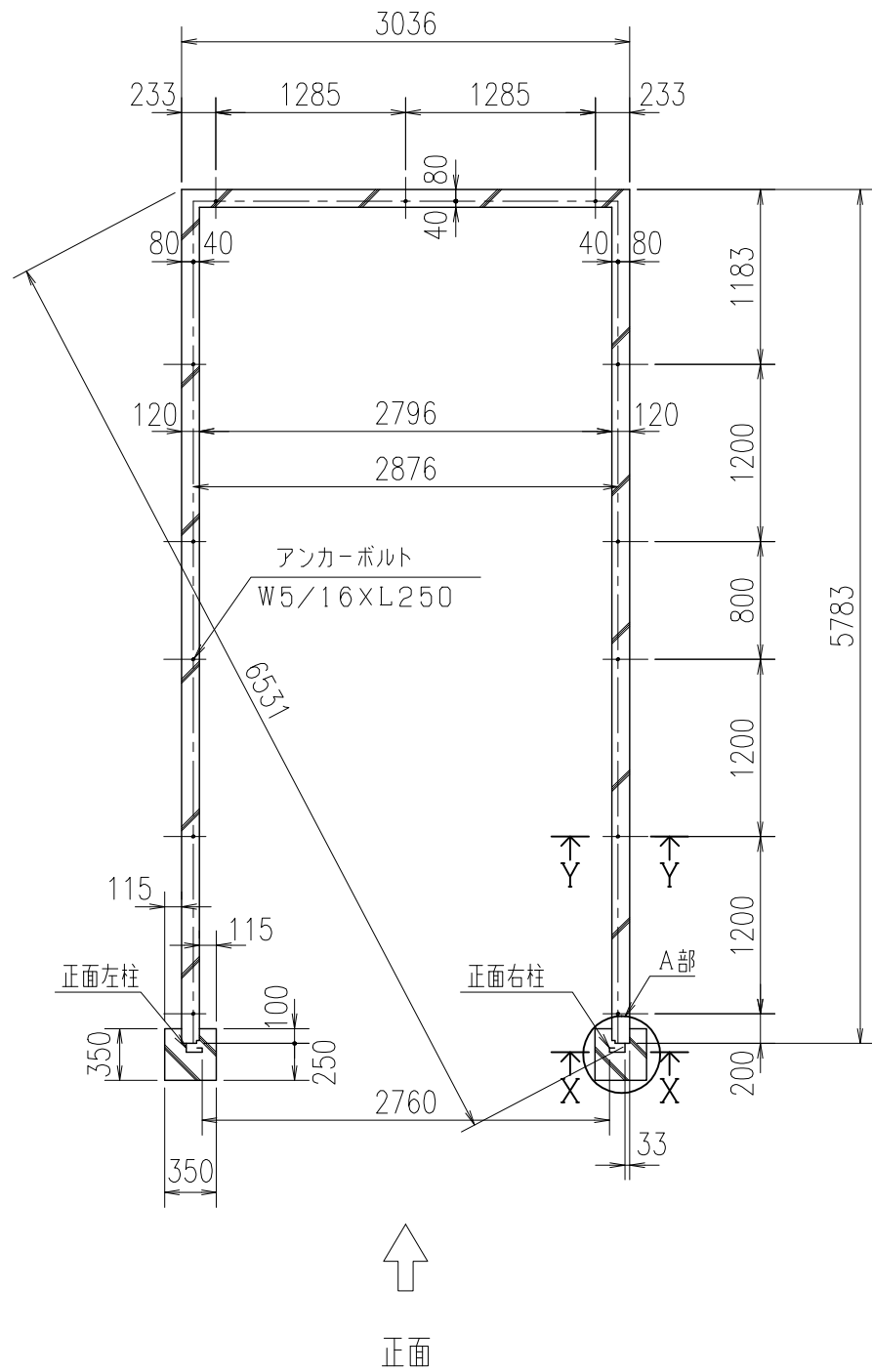
基礎平面図 S = 1 / 50
