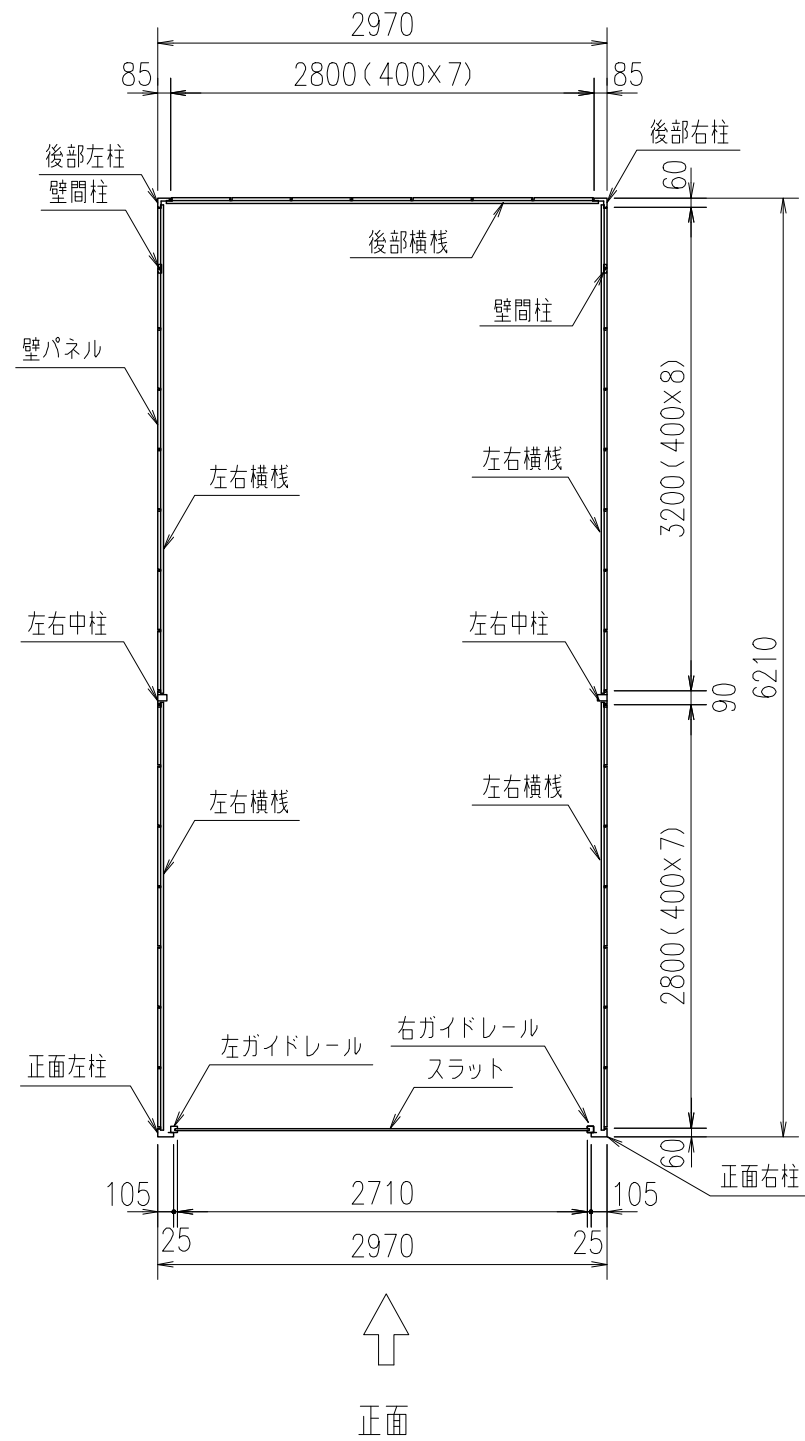
平面断面図
