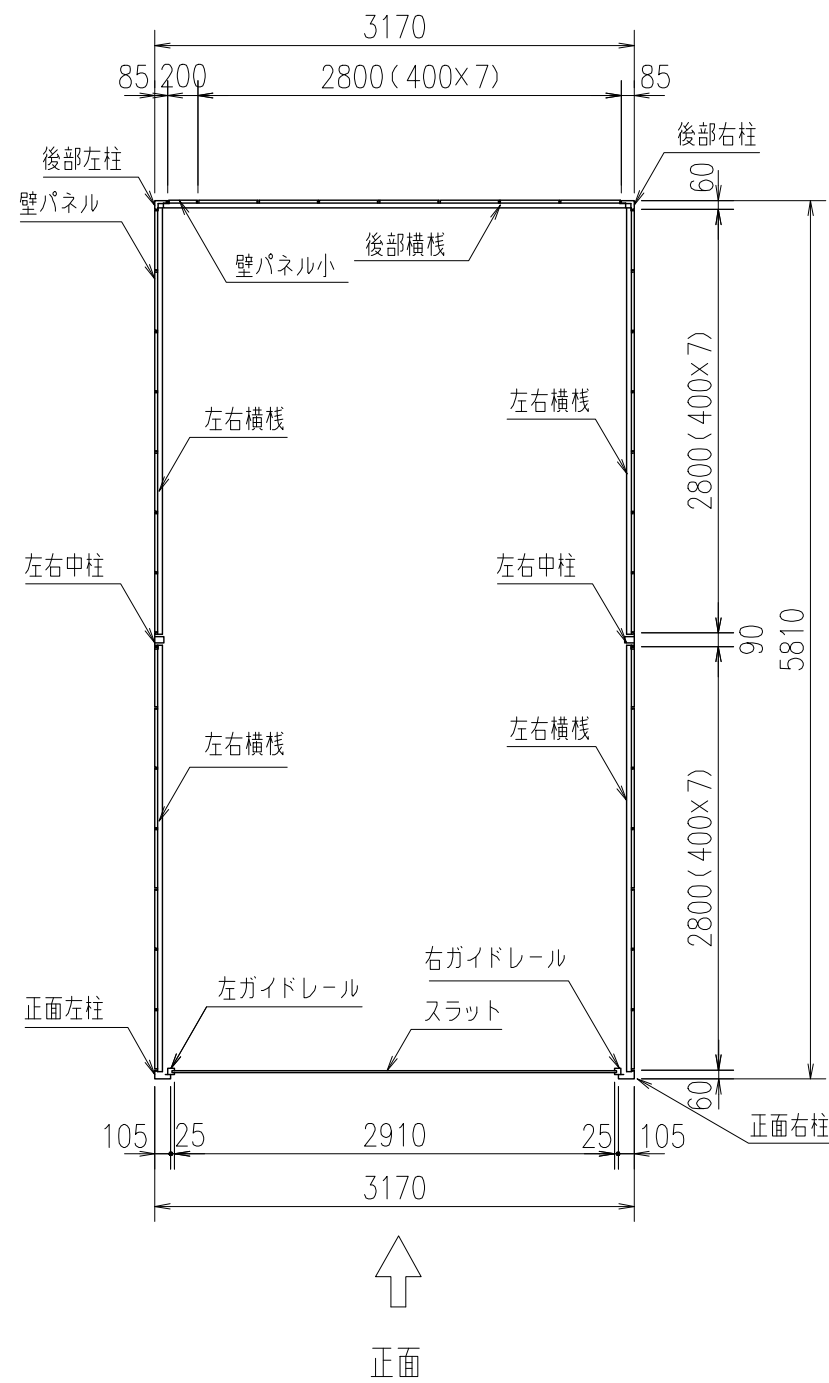
平面断面図
