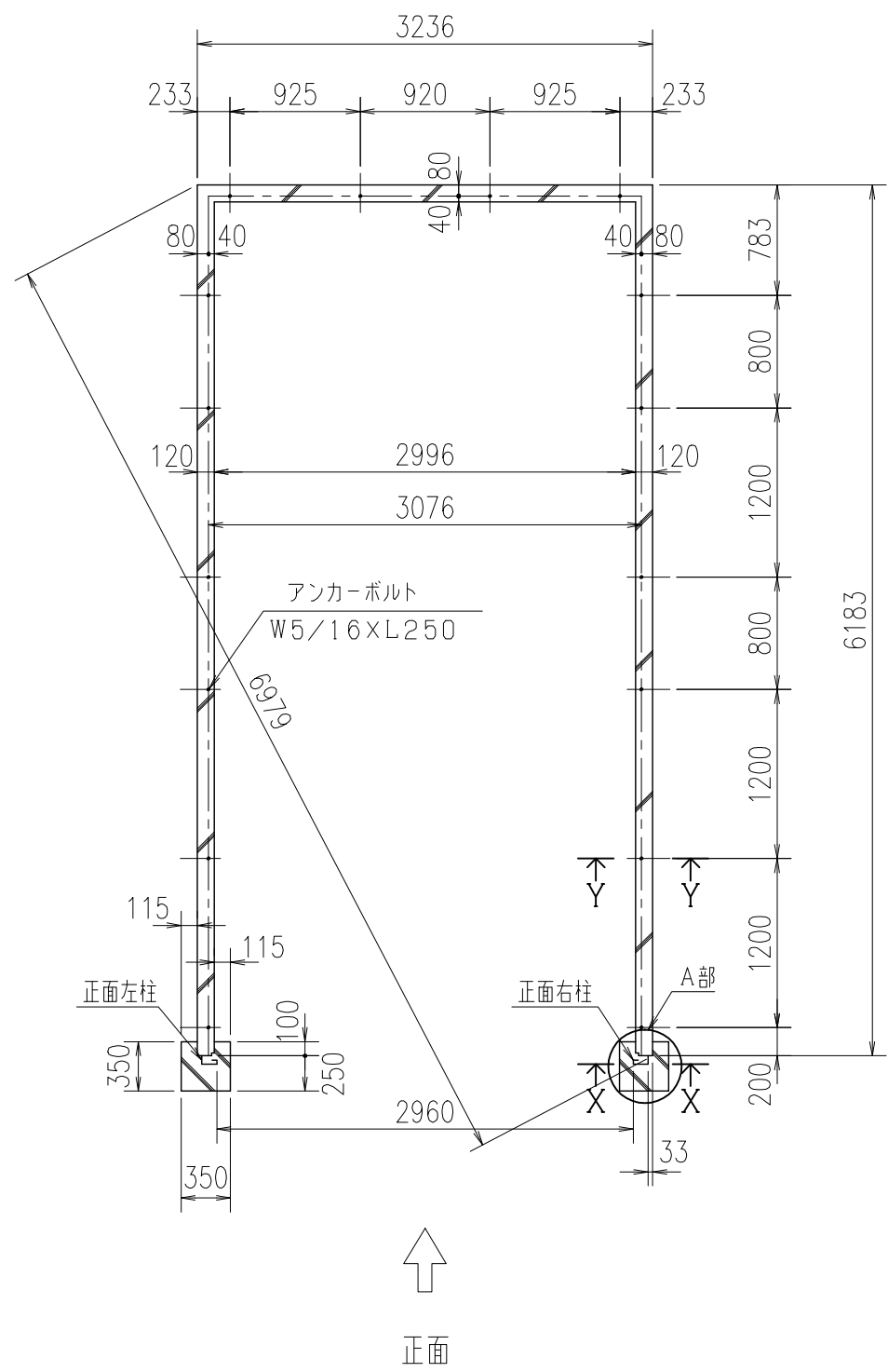
基礎平面図 S = 1 / 50
