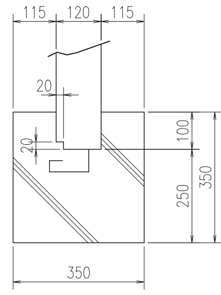
A部詳細 S = 1 / 10
