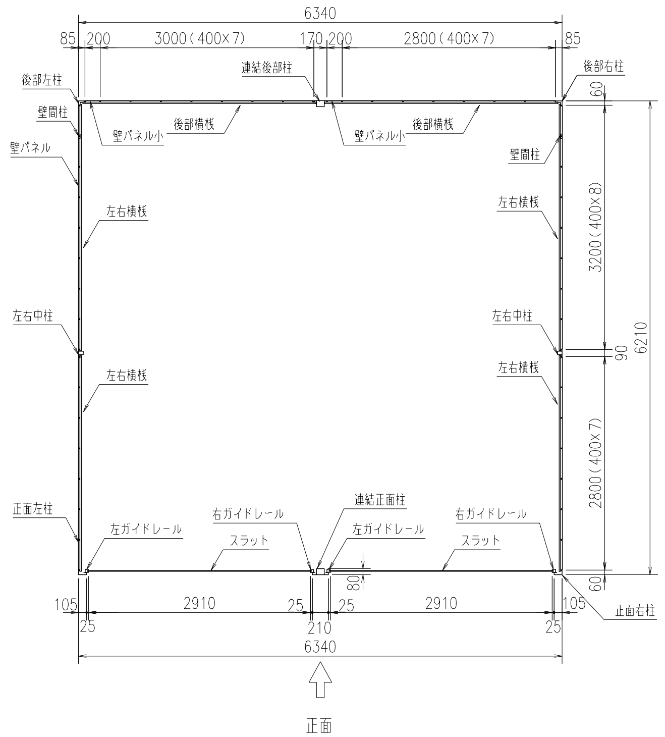
平面断面図
