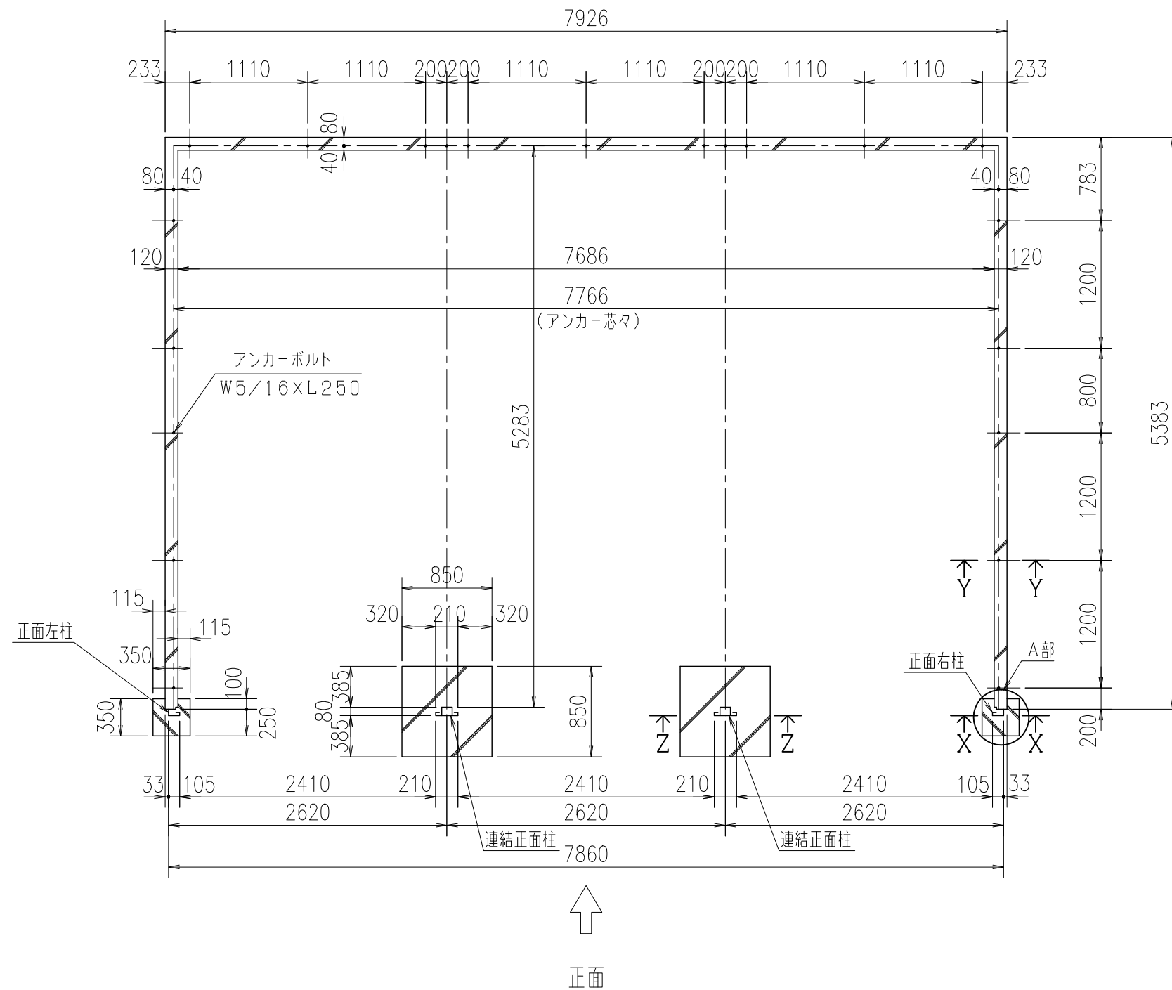
基礎平面図
