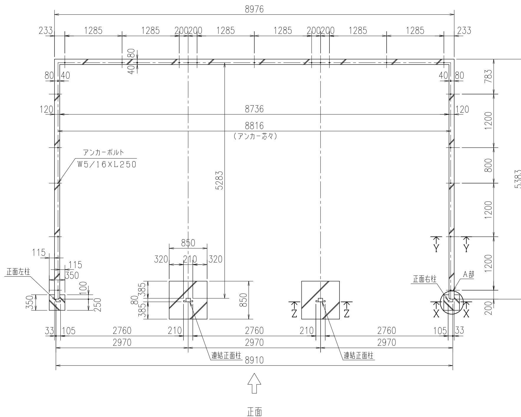
基礎平面図
