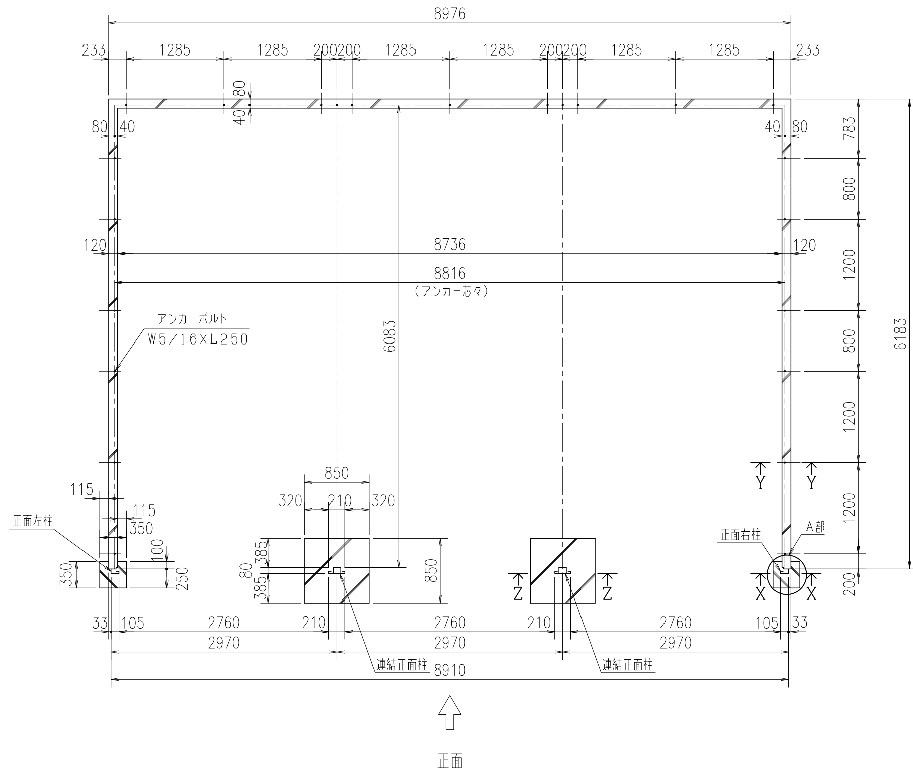
基礎平面図
