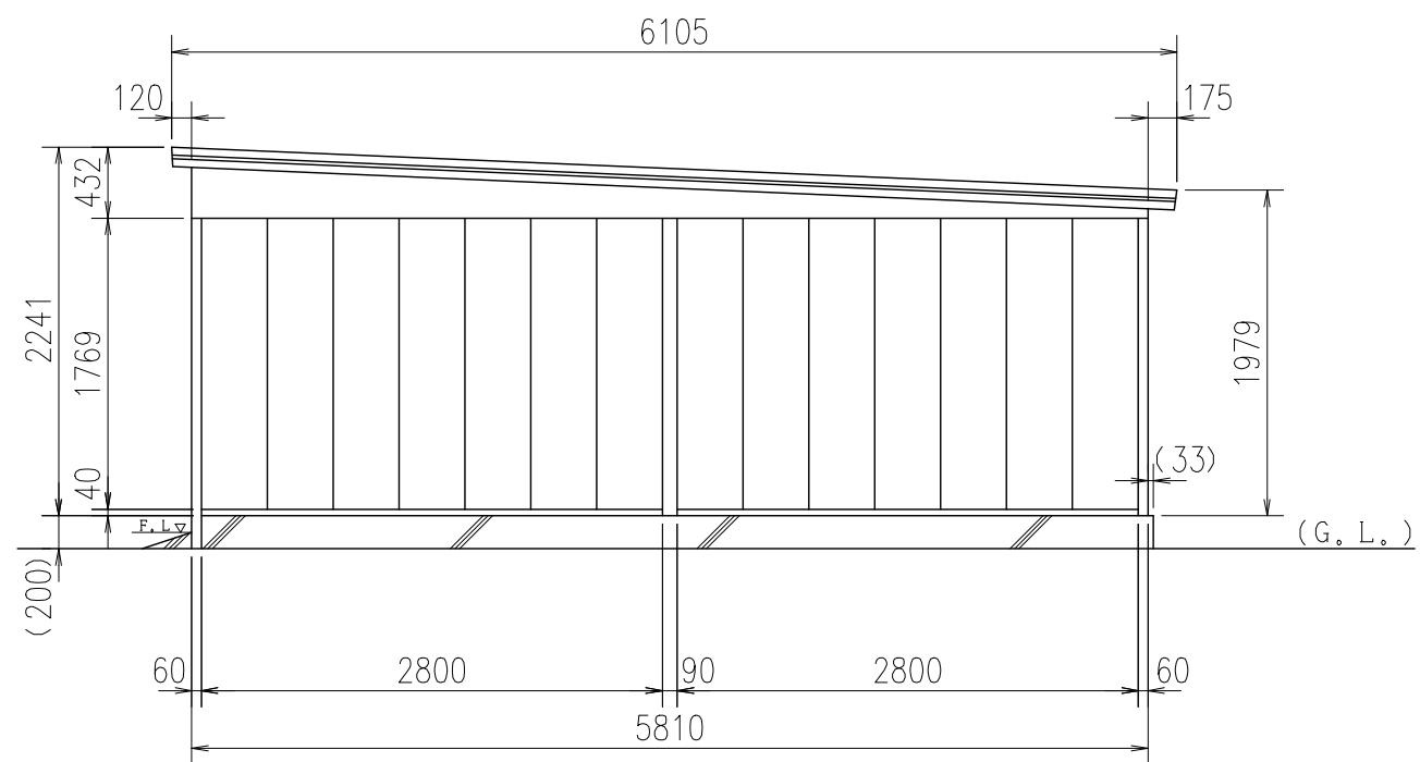
側面図
