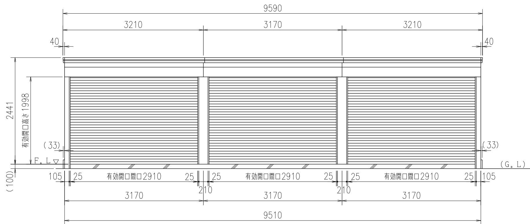
正面図
