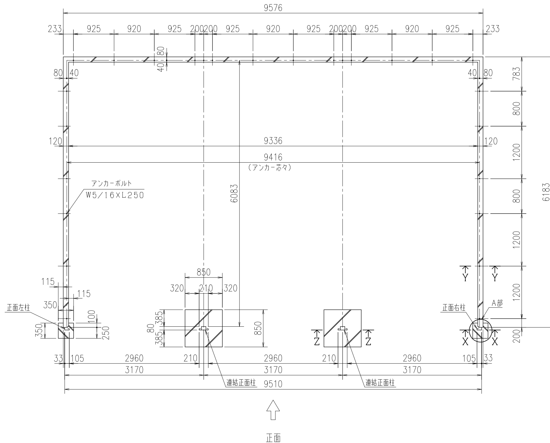
基礎平面図
