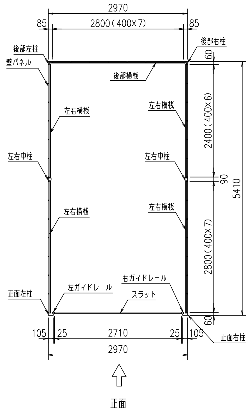
平面断面図
