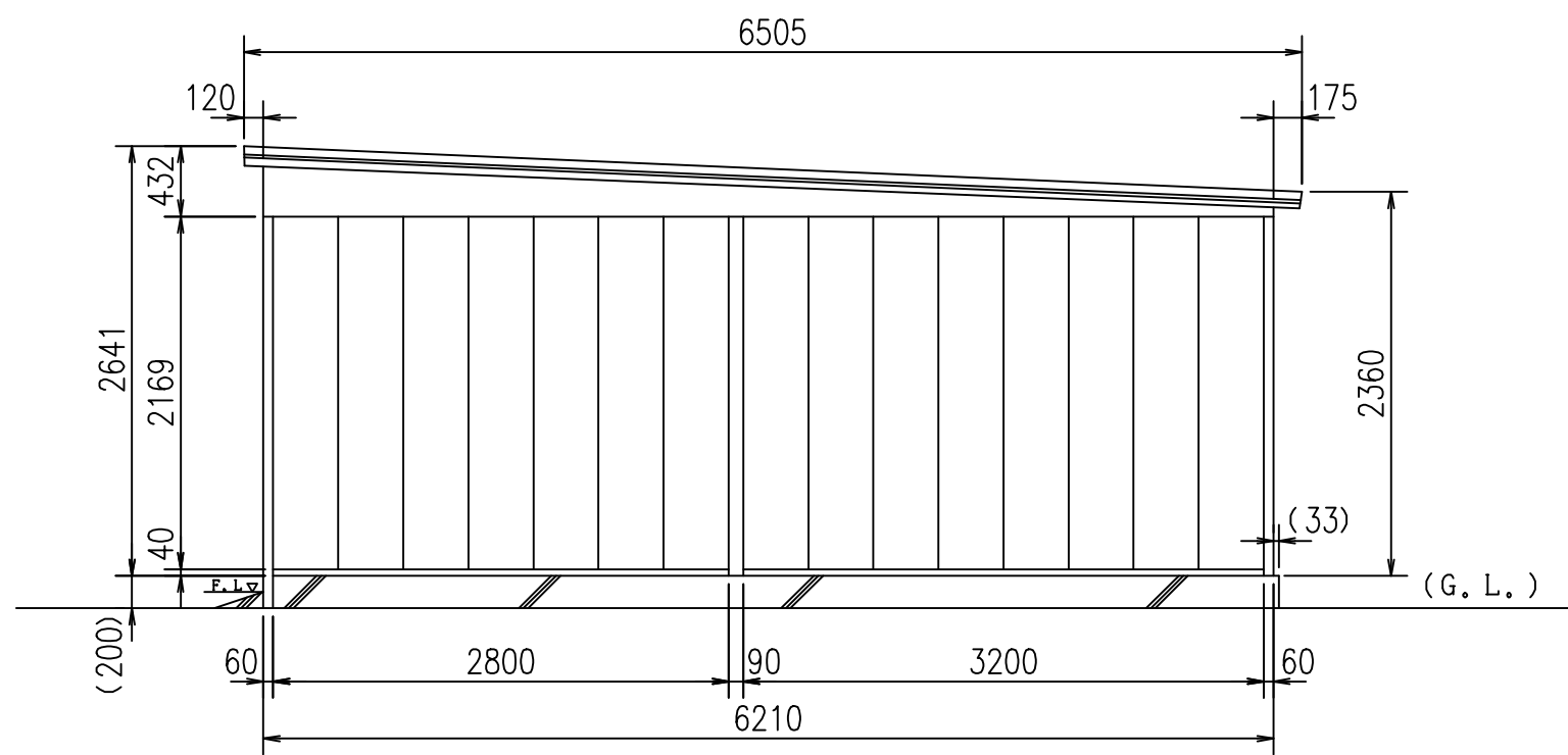
側面図
