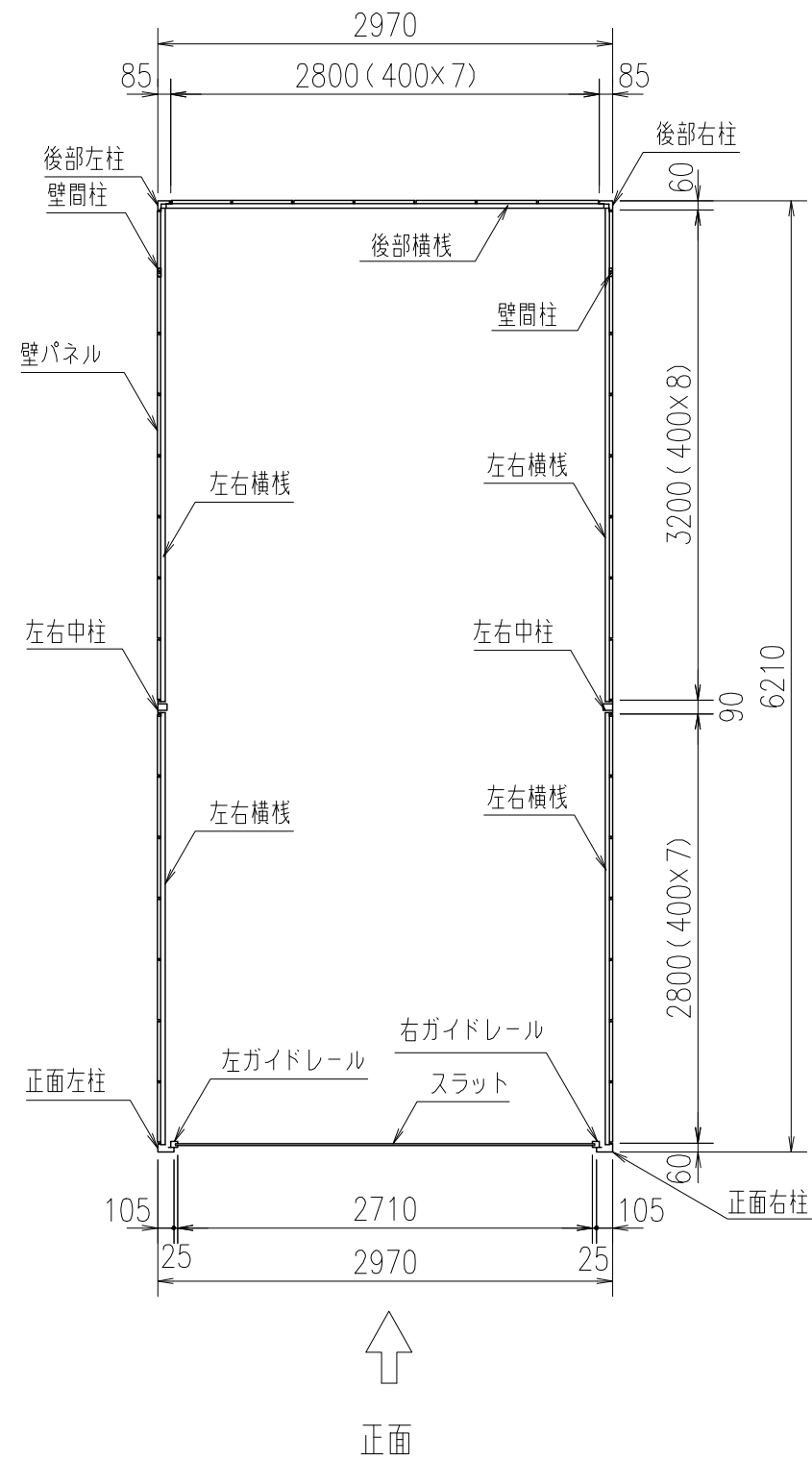
平面断面図
