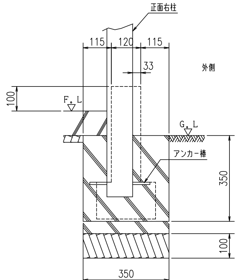
X-X断面図 (正面右柱基礎) S = 1 / 10
