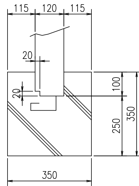
A部詳細 S = 1 / 10
