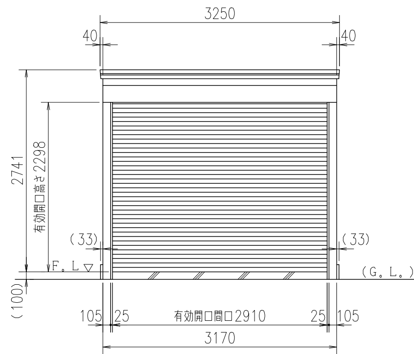
正面図
