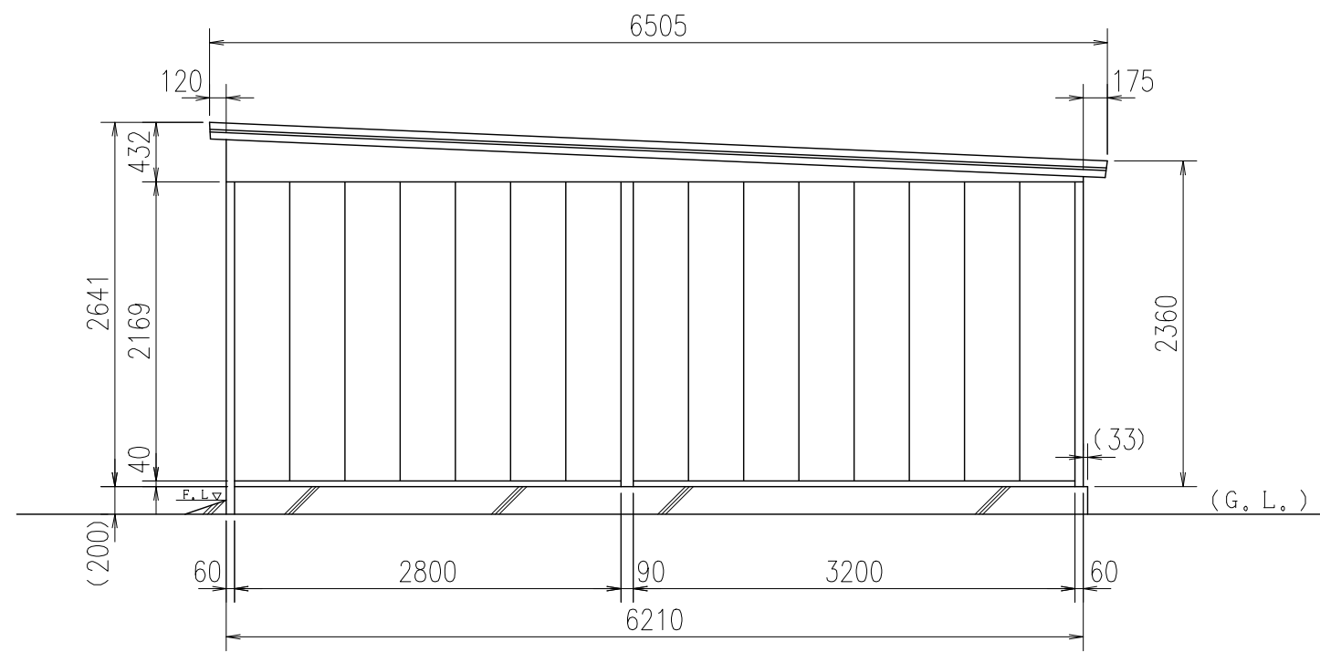
側面図
