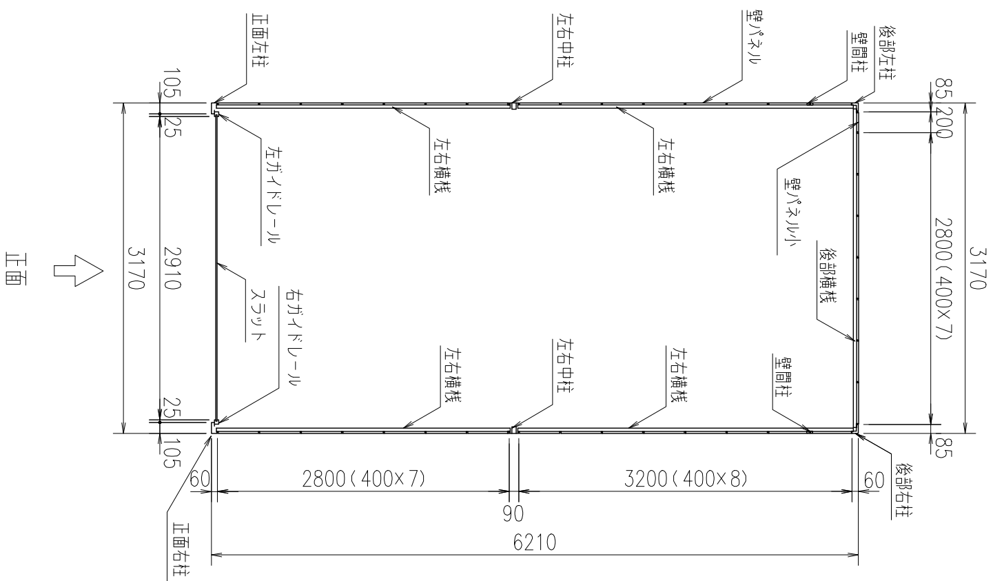
平面断面図
