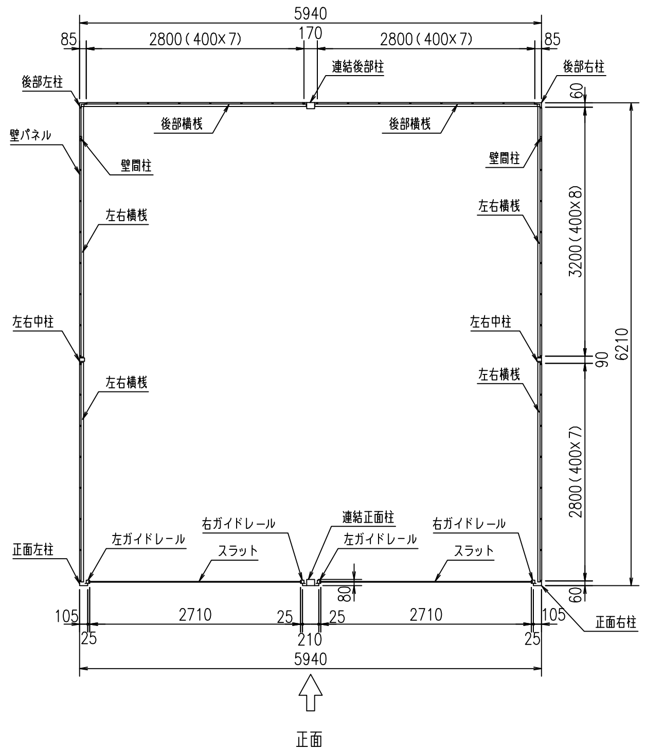
平面断面図
