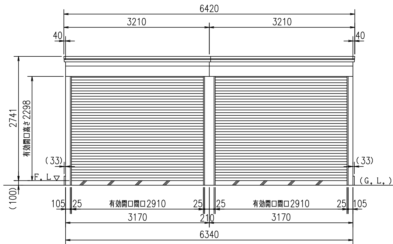
正面図
