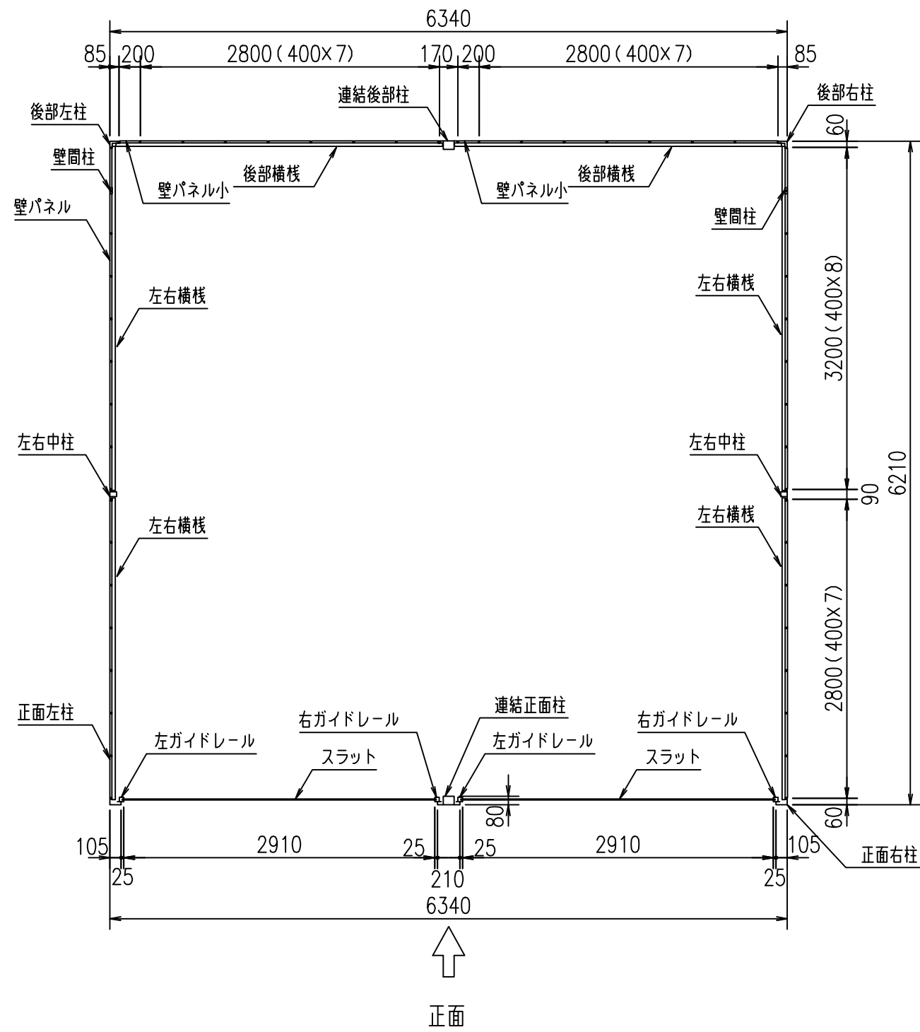
平面断面図
