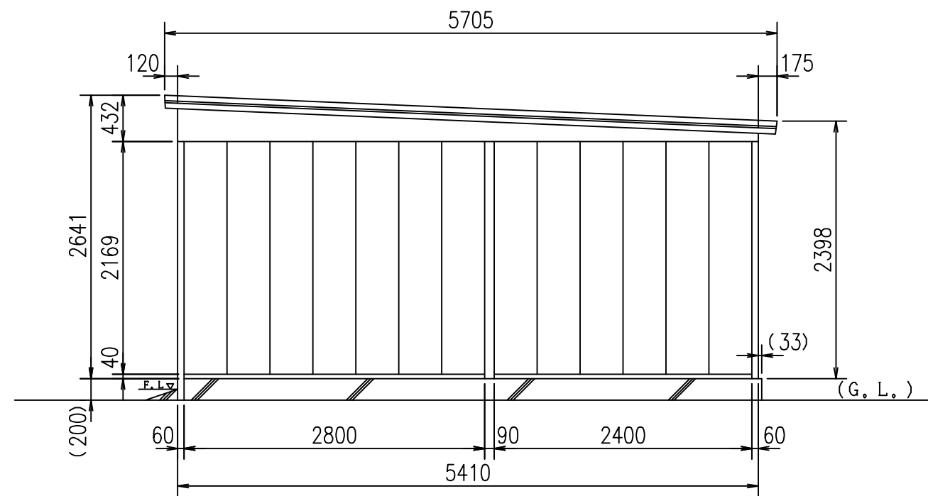
側面図
