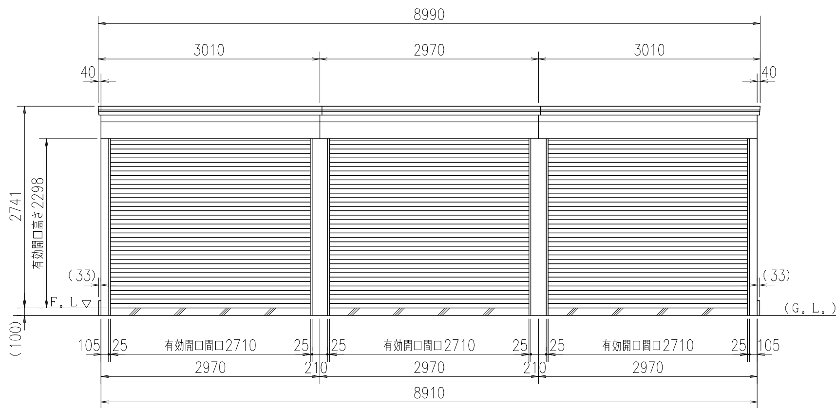
正面図
