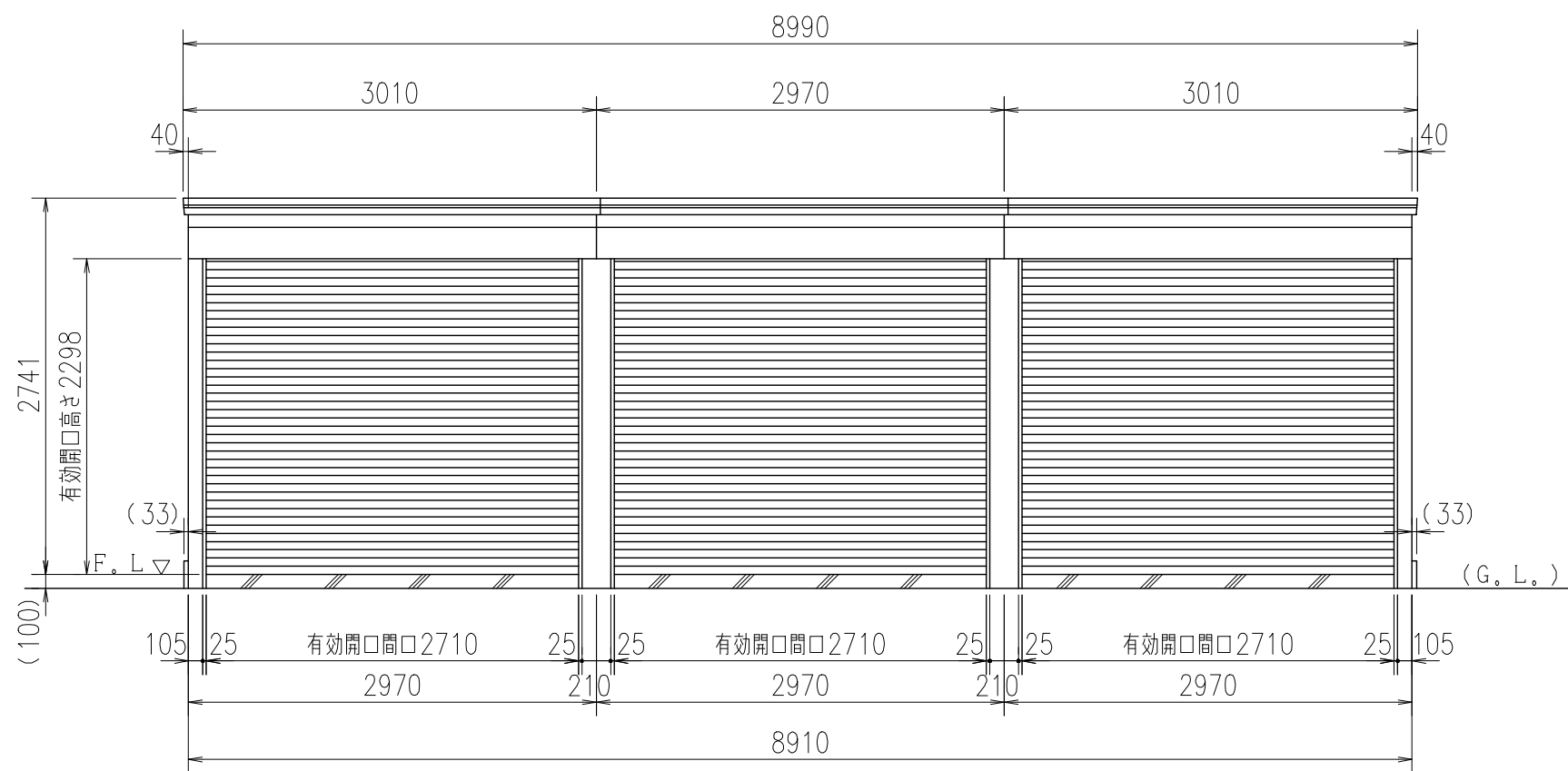
正面図
