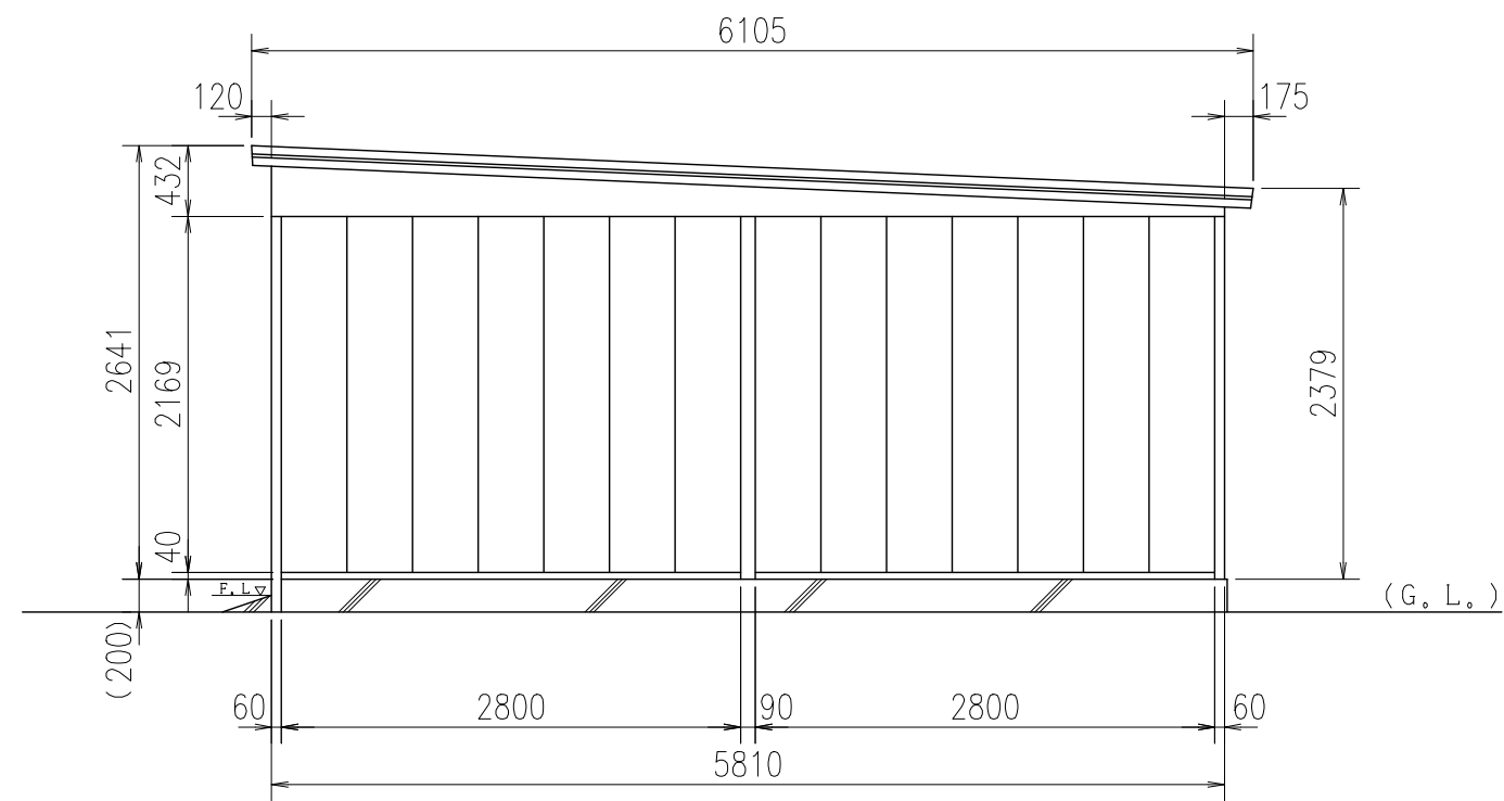
側面図
