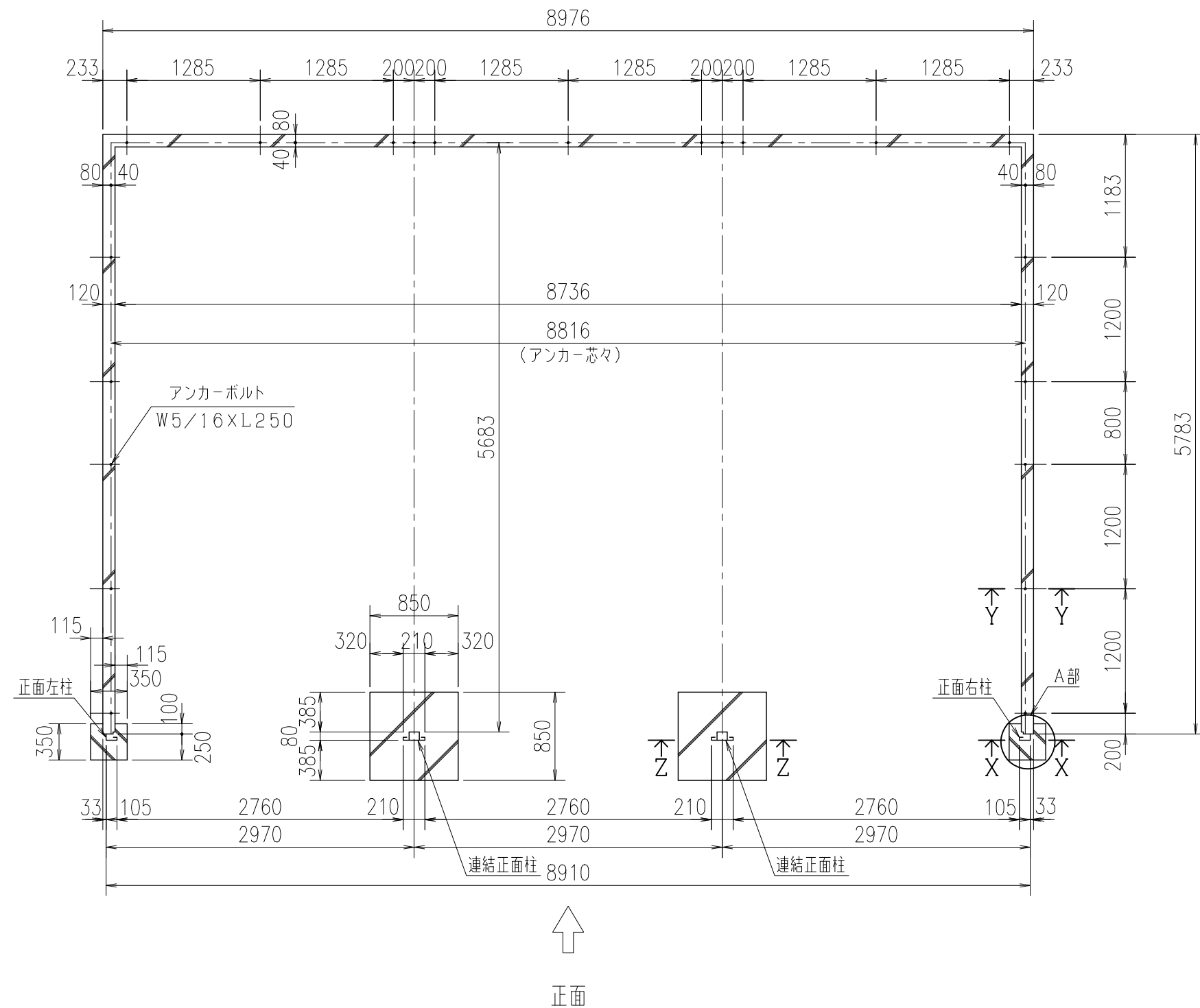
基礎平面図
