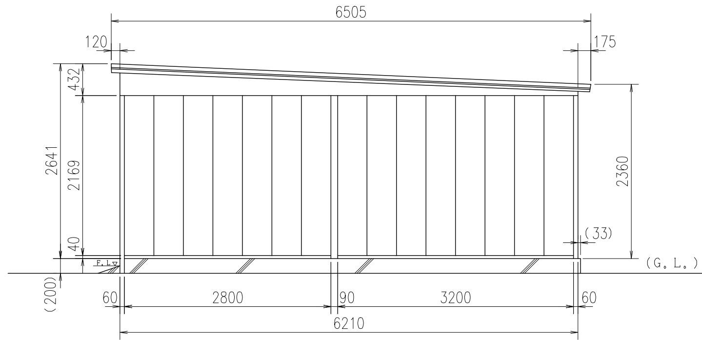
側面図
