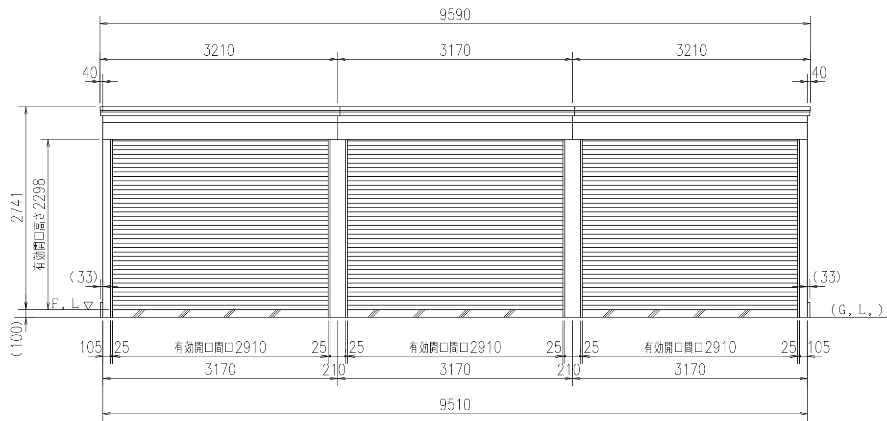
正面図
