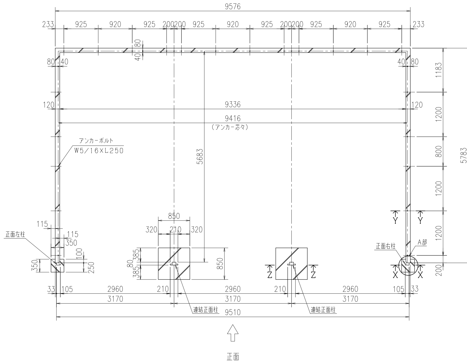
基礎平面図
