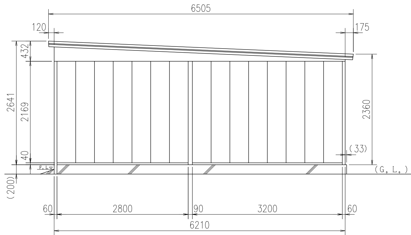
側面図
