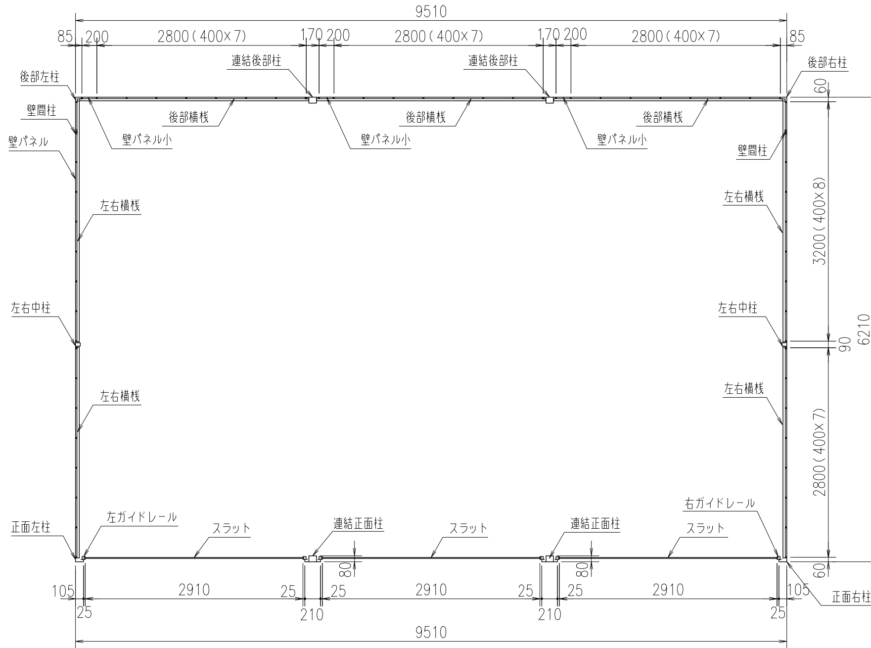
↑ 正面 平面断面図
