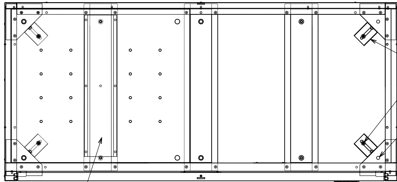
2-底板 (取り外し可能) A-A断面図 (右側底板を取り外した状態)
