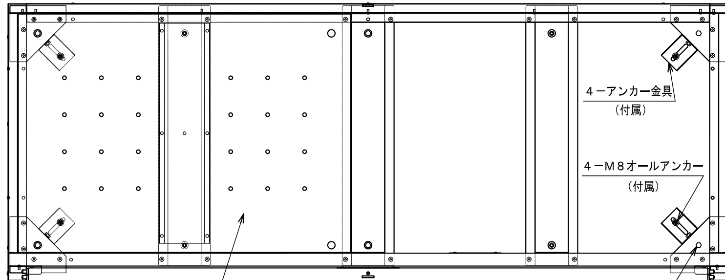
6-レベル調整用ボルト (M8×40ステンレス六角ボルト) (M8×70ステンレス六角ボルト)
