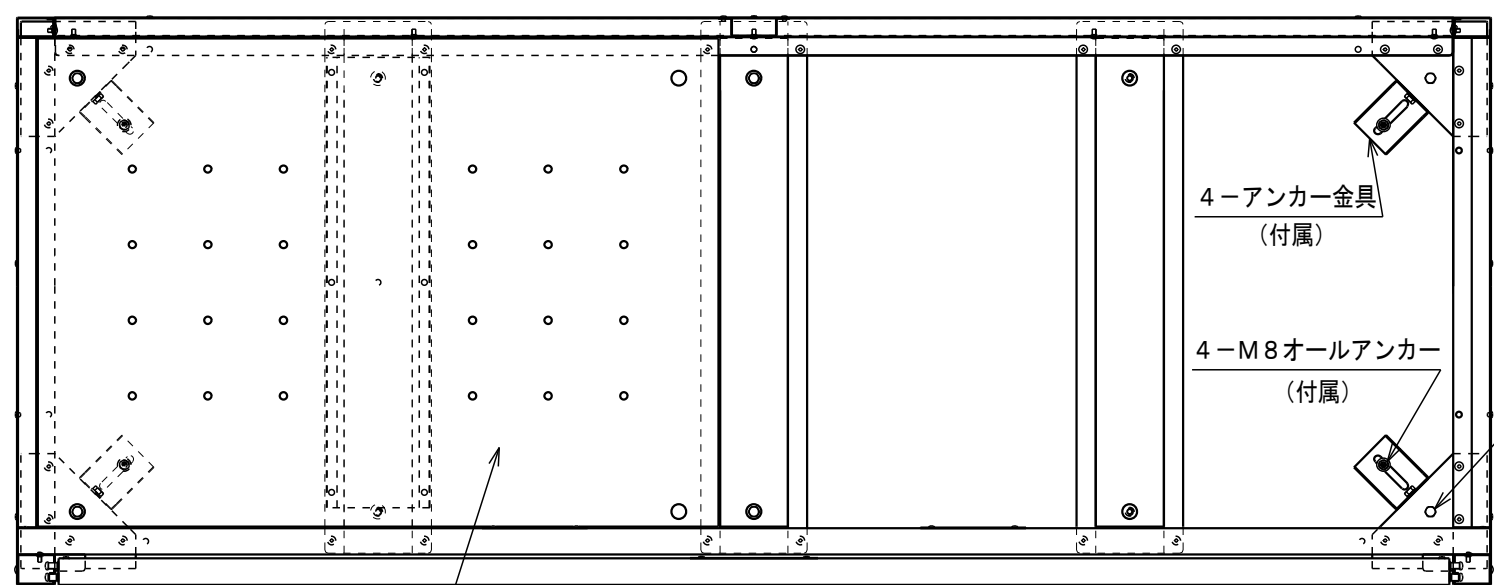
2-底板 (取り外し可能) A-A断面図 (右底板を取り外した状態) 上扉取手 上扉
