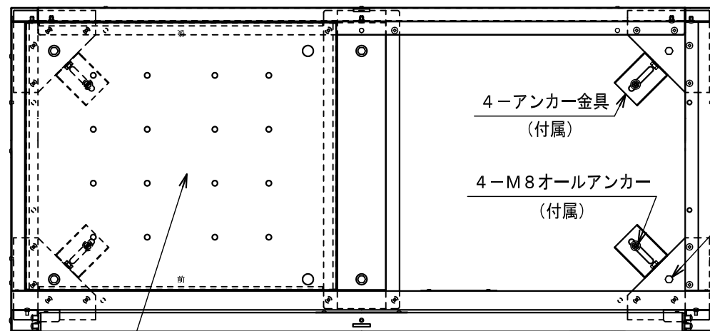
2-底板 (取り外し可能) A-A断面図 (右側底板を取り外した状態)
