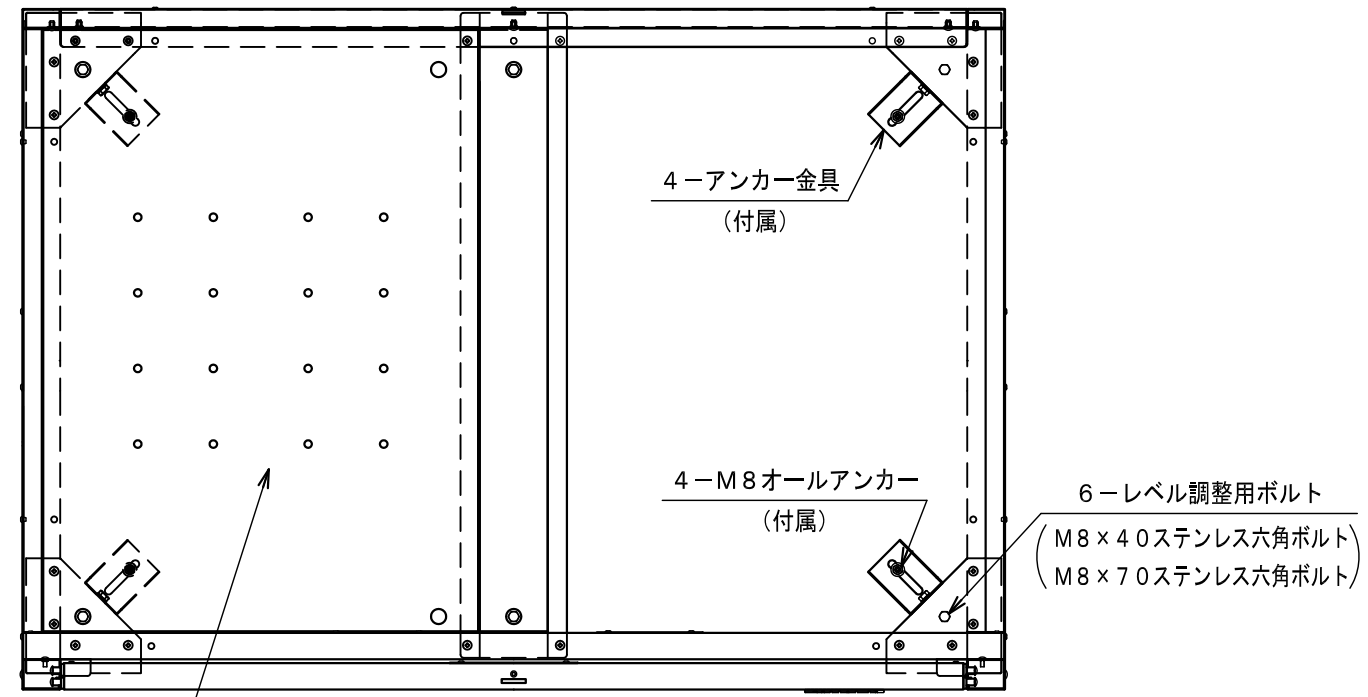
2-底板 (取り外し可能) A-A断面図 (右側底板を取り外した状態)
