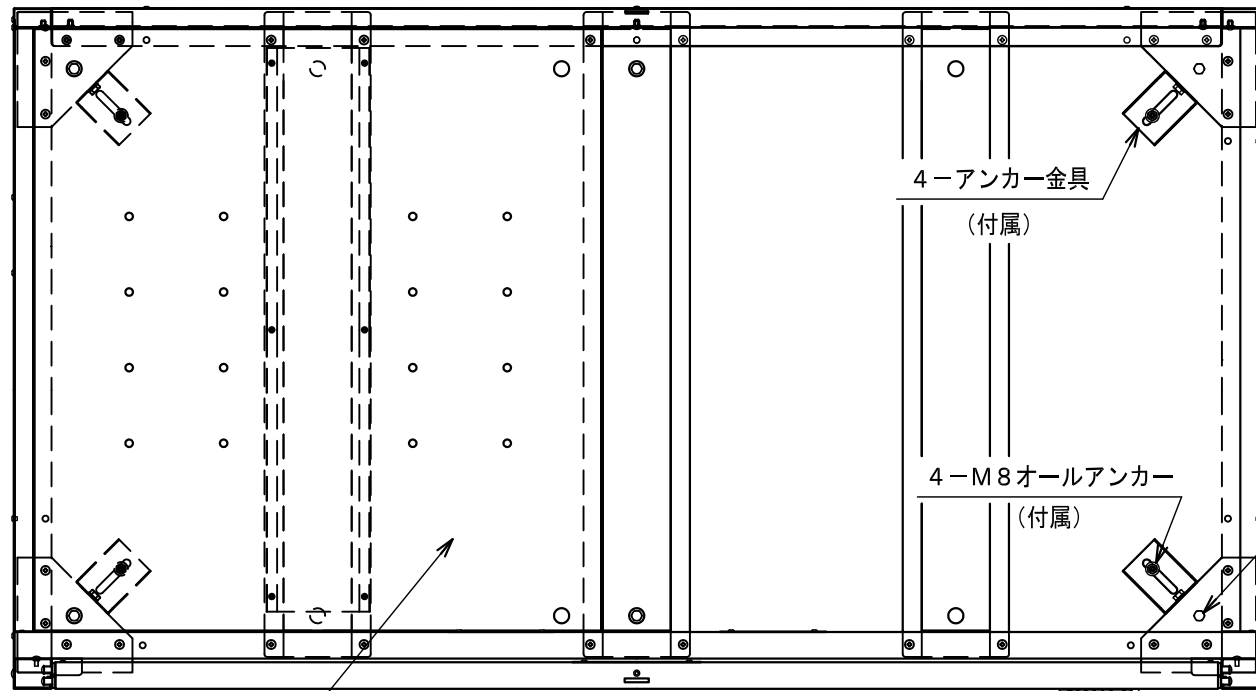
2-底板 (取り外し可能) A-A断面図 (右側底板を取り外した状態)
