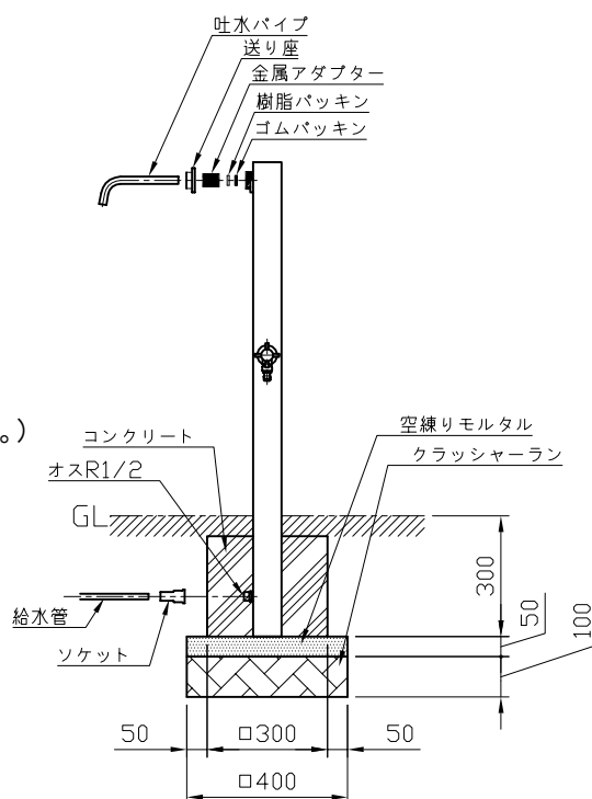
参考施工図
