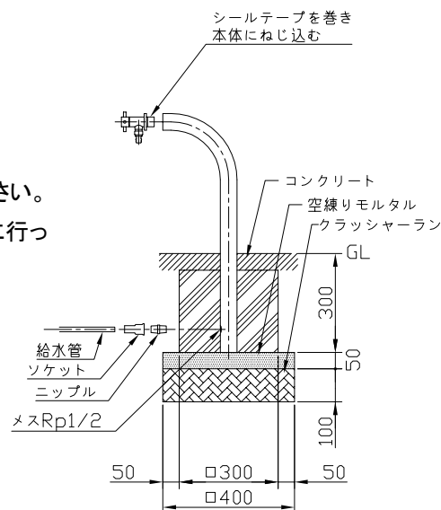
参考施工図
