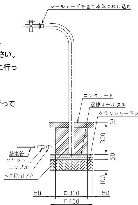
参考施工図
