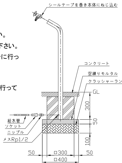
参考施工図
