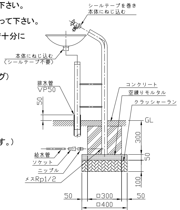
参考施工図
