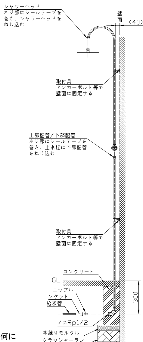
参考施工図
