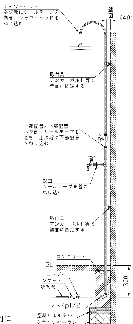
参考施工図
