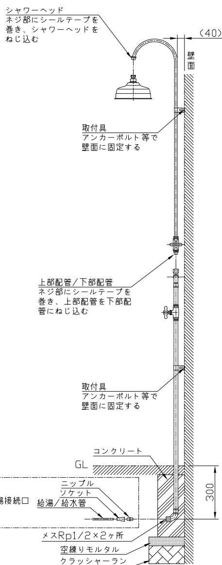
参考施工図
