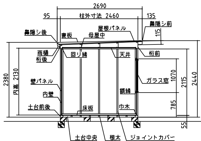
断面図
