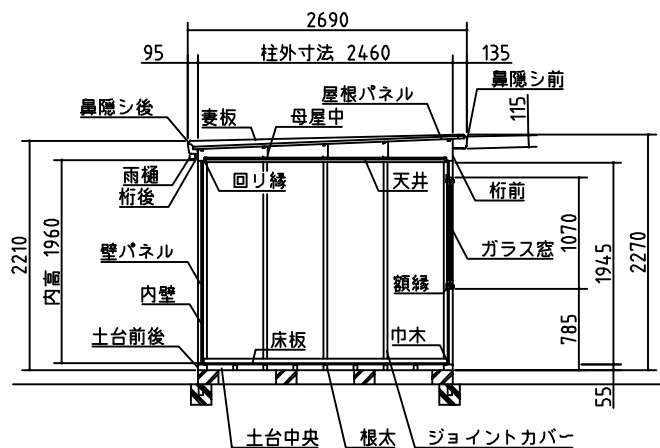
断面図
