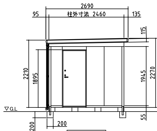
側面図
