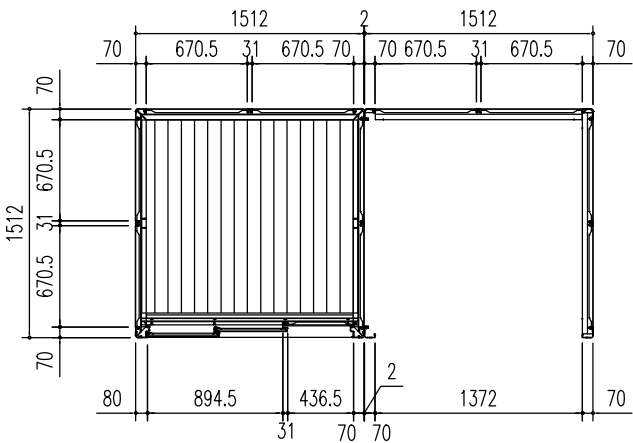
平面図 (S = 1/50)
