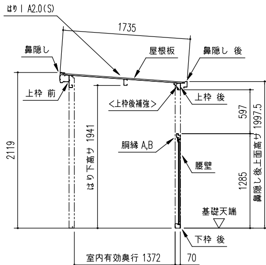
[オープン部] 矩計図 (S = 1/50)
