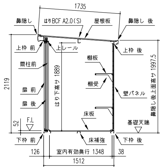
[物置部] 矩計図 (S = 1/50)
