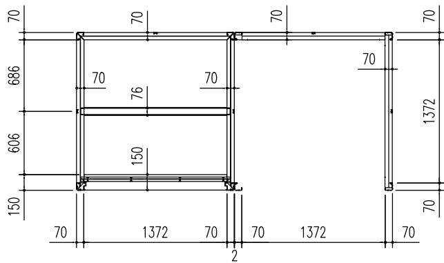
床伏図 (S = 1/50)
