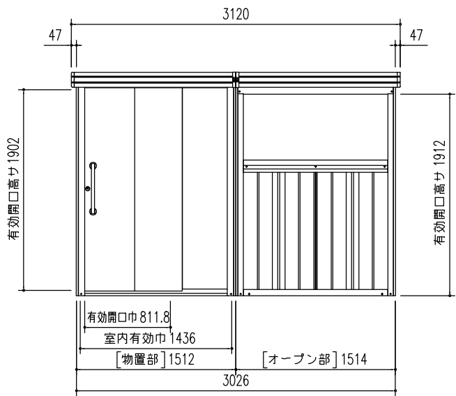
正面立面図 (S = 1/50)
