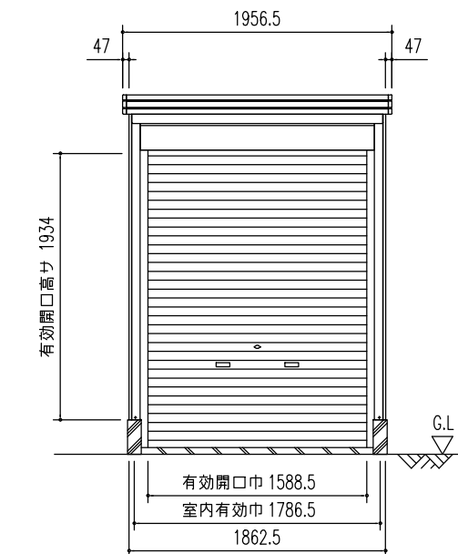
正面立面図 (S=1/50)
