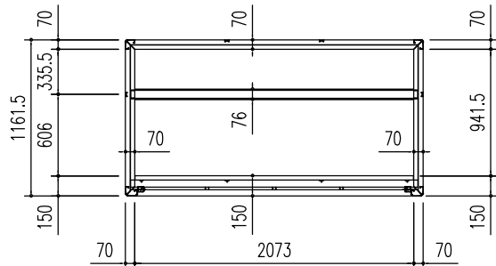
床伏図 (S = 1/50)
