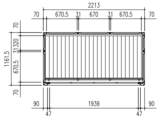
平面図 (S = 1/50)
